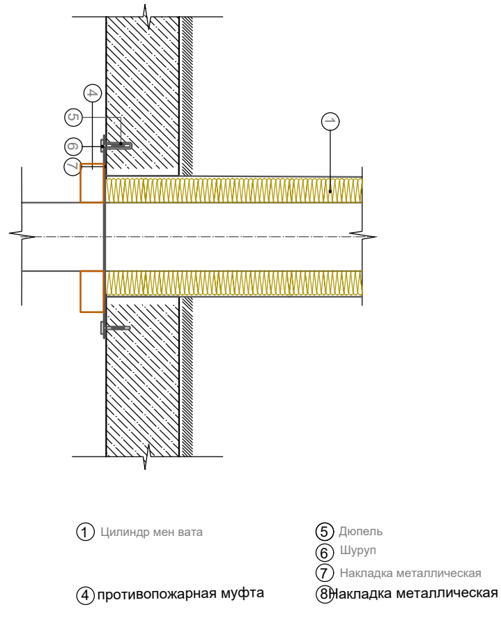
Типовой узел прохода трубопровода через стены
