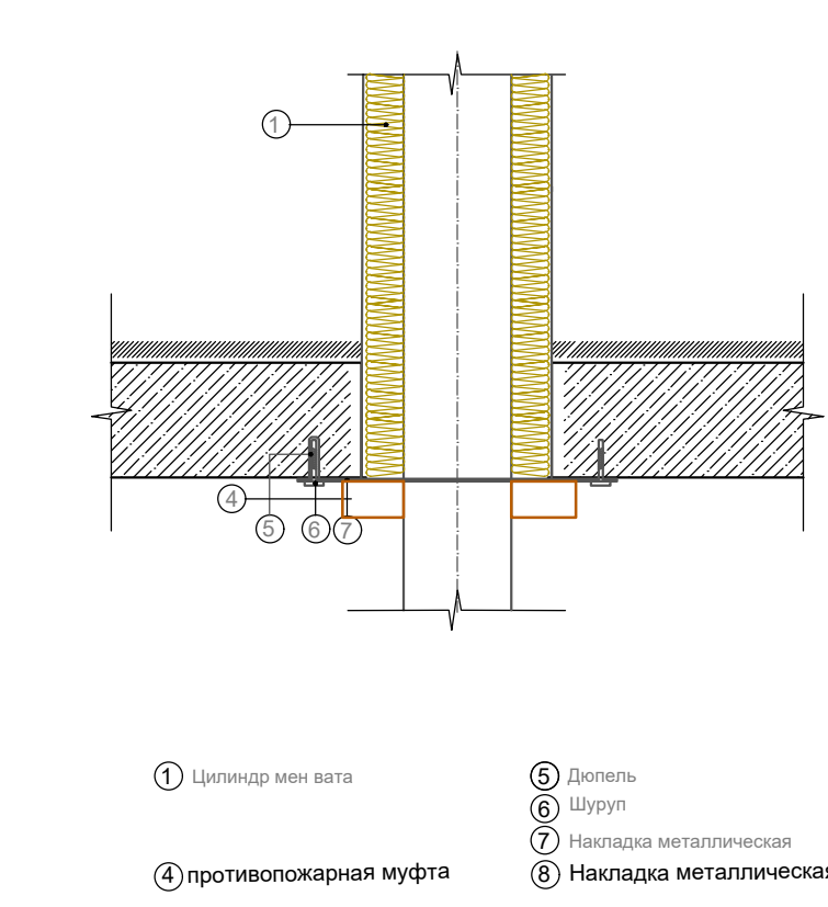
Типовой узел прохода трубопровода через перекрытие
